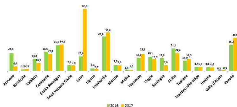
Potenza connessa per regione [MW]
