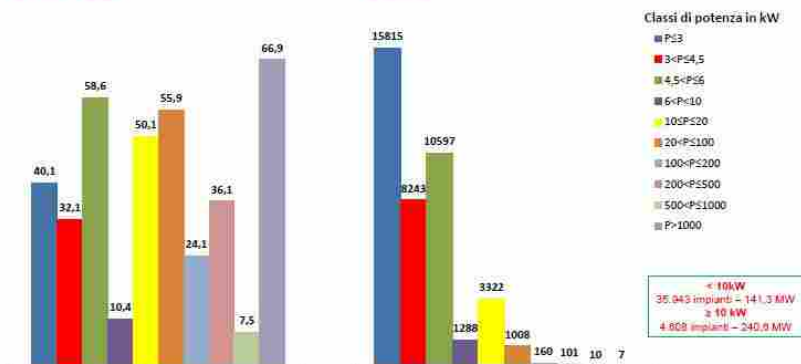
Potenza connessa per classi di potenza nel 2017 [MW]
