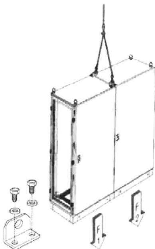
Figura 3 - Attraverso squadrette di sollevamento per un'ottimale distribuzione del carico per armadi accoppiati e movimentati via cavi di sollevamento.
