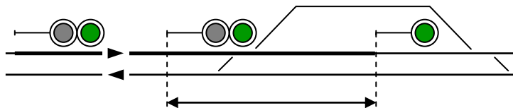
Transito su binario di corretto tracciato
