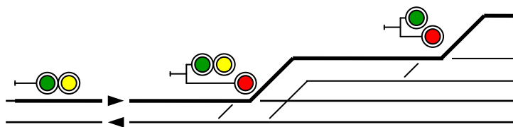
Transito per itinerario con due diramazioni successive aventi entrambe lo scambio disposto per il ramo deviato (riduzione di velocità a 30 km/h).
