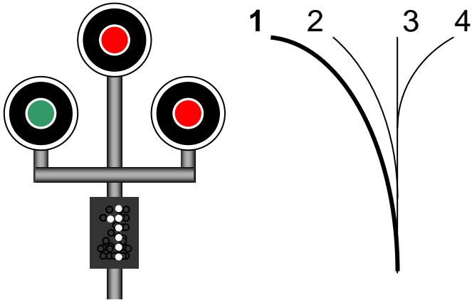
Segnale a candeliere integrato da indicatore, a via libera per la direzione 1.
