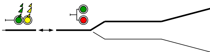
Transito su bivio simmetrico (riduzione di velocità a 60 km/h)
