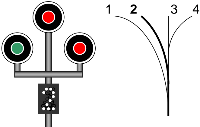
Segnale a candeliere integrato da indicatore, a via libera per la direzione 2.
