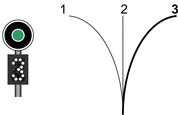
Segnale a luce unica integrato da indicatore, a via libera per la direzione 3.
