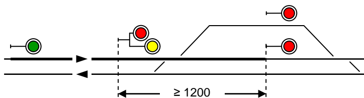
Ingresso in binario di corretto tracciato e fermata in stazione quando la distanza fra il segnale di protezione e il segnale di partenza sia uguale o superiore a m. 1200.
