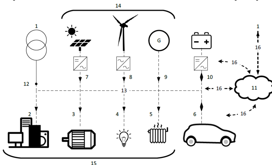
Figura 15 -PEI: schema di principio (fonte CEI 64-8/8-2)
