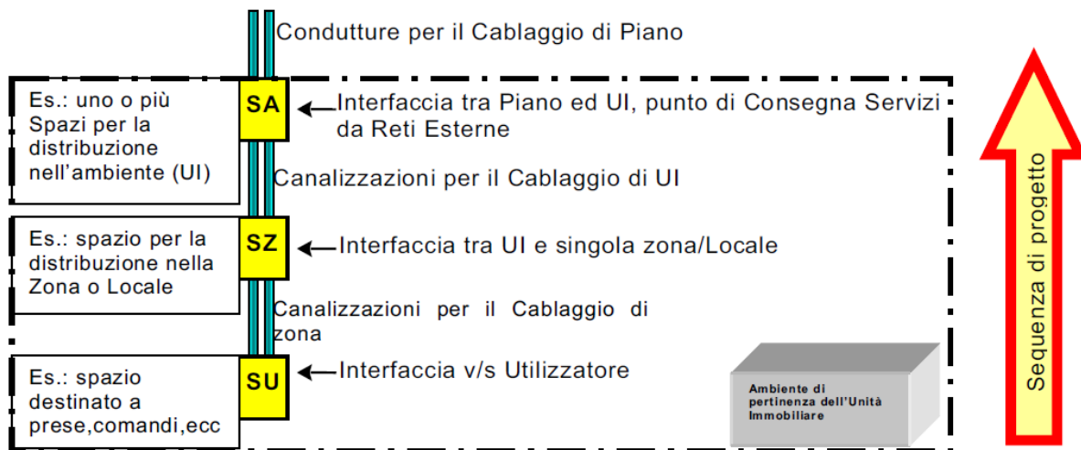
Figura 10 Schema di principio di una infrastruttura integrata per impianti elettrici ed elettronici
