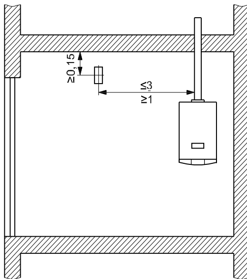
Tipica installazione del rivelatore per gas monossido di carbonio CO
