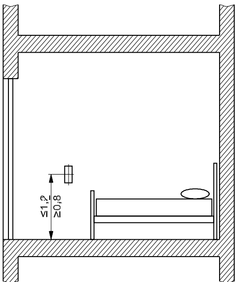
Tipica installazione del rivelatore per gas monossido di carbonio CO
